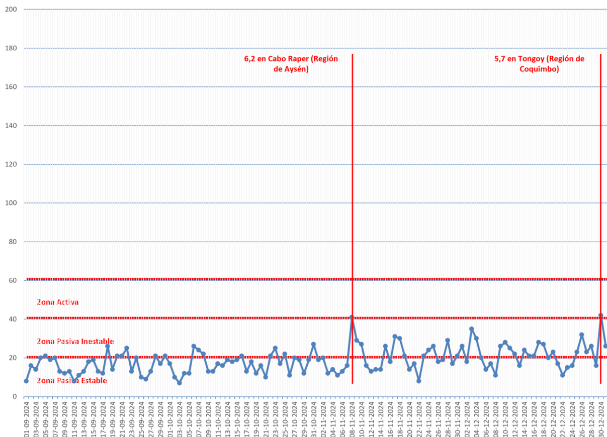
SISMOS POR DIA EN CHILE (Sep, Oct, Nov, Dic del 2024)
